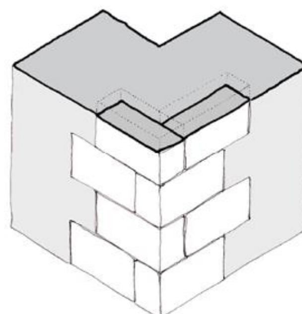
Λαξευτοί ακρογωνιαίοι λίθοι.
