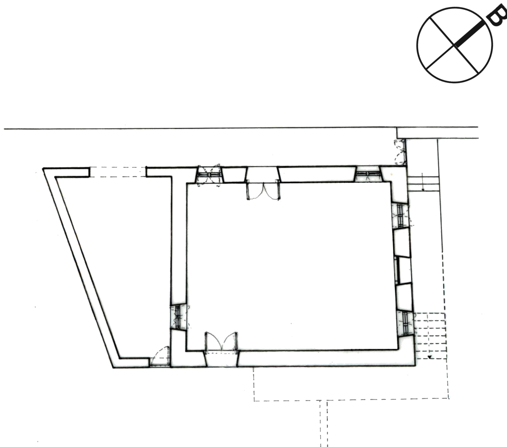
ΚΑΤΟΨΗ ΙΣΟΓΕΙΟΥ
